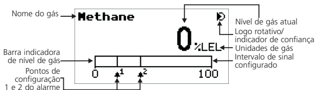
Diagrama 18: Tela de status de gás
