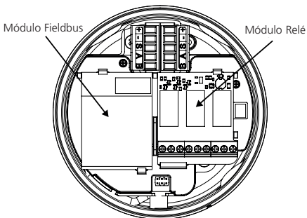
Diagrama 3: Módulo de relés e o espaço/conector para o módulo Foundation Fieldbus
