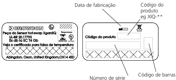
Diagrama 6: Etiquetas do módulo sensor
