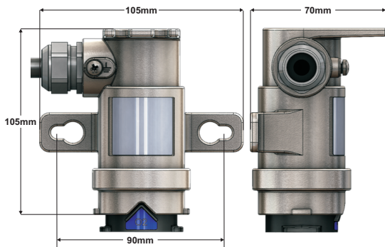
Diagrama 9: Dimensões do alojamento do sensor remoto
